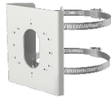
DS-1275ZJ-S-SUS Vertikale Masthalterung
